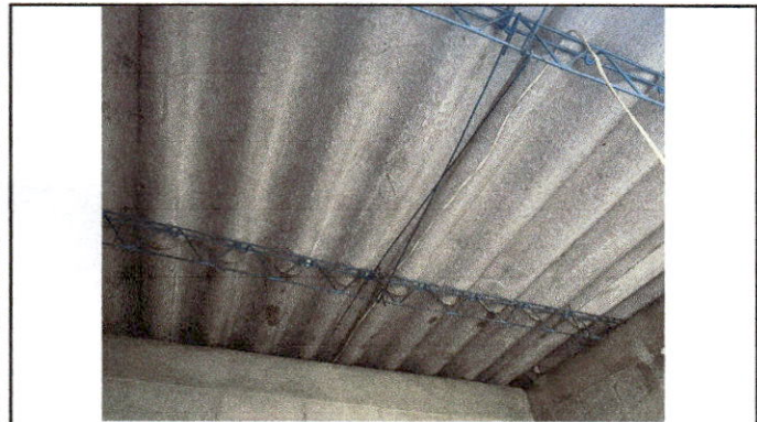
Foto 3: Módulo A, estructura metálica en mal estado
