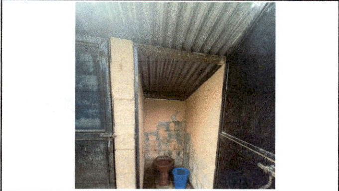
Foto 9: Módulo B, lámina y estructura portante en letrinas en mal estado
